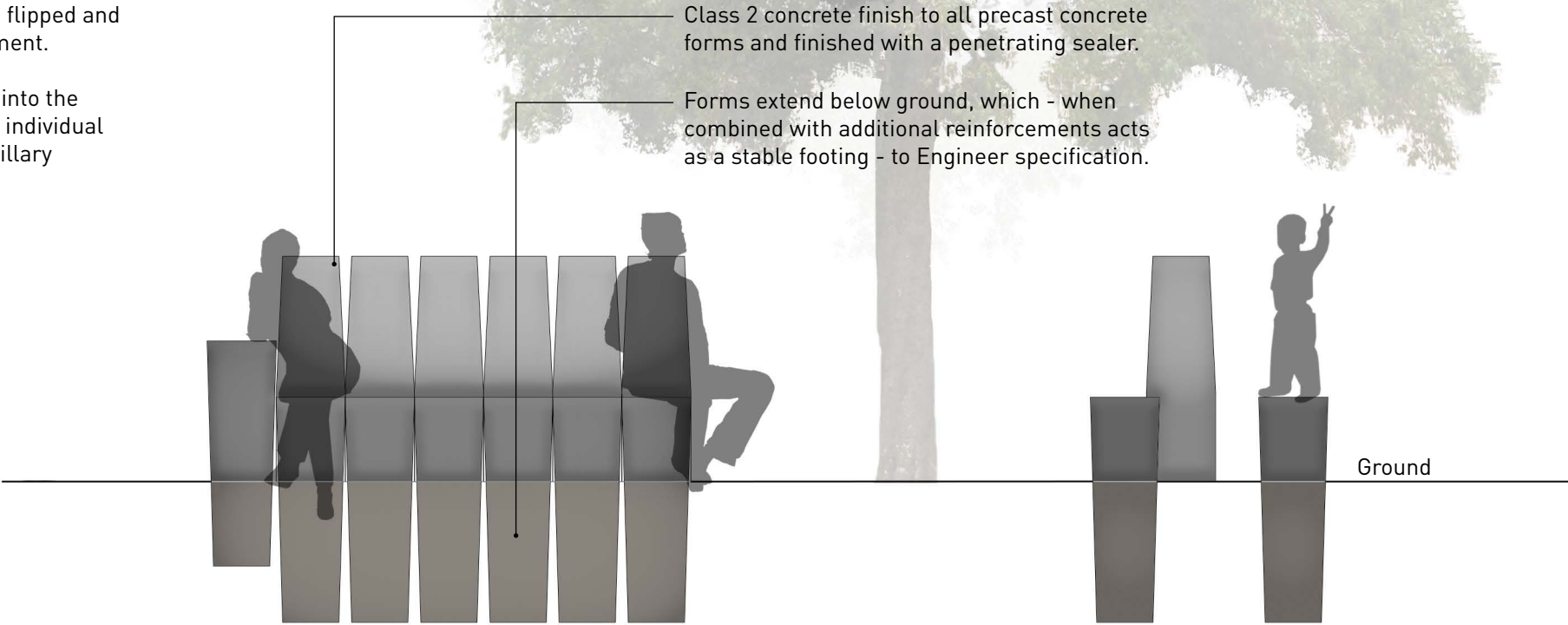
ELEVATION
